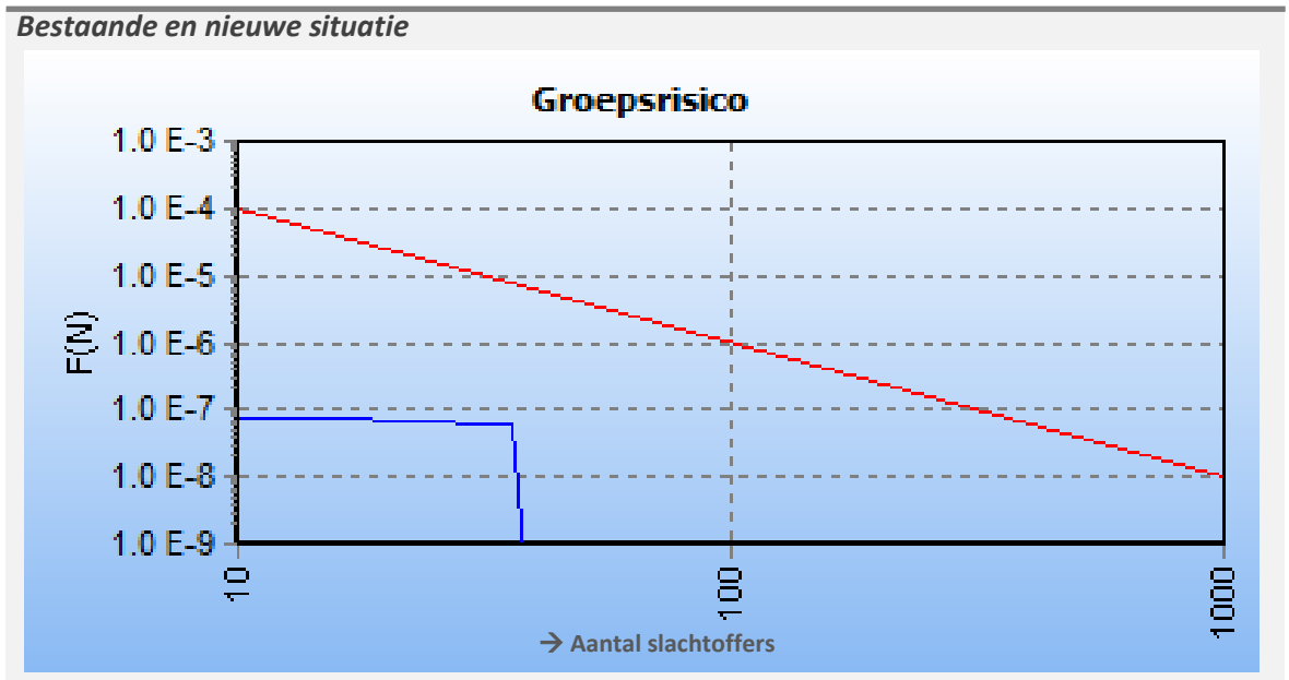
Figuur 6.3 FN curve voor buisleiding A-637 van Gasunie voor de kilometer tussen stationing 1430.00 en 2430.00 (bestaande situatie en stationing 1680.00 en 2680.00 (nieuwe situatie)
