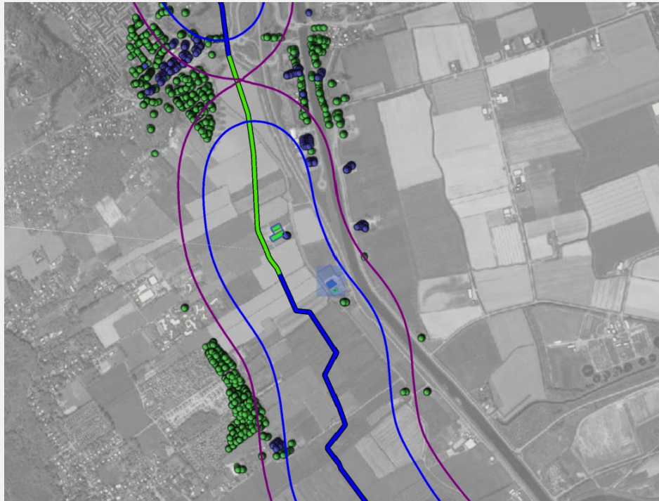
Nieuwe situatie A-637
