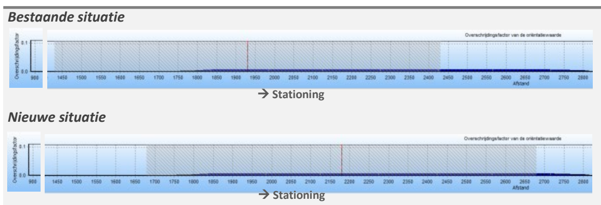
Figuur 6.2 Groepsrisico screening voor A-637 van Gasunie bestaand en nieuw
