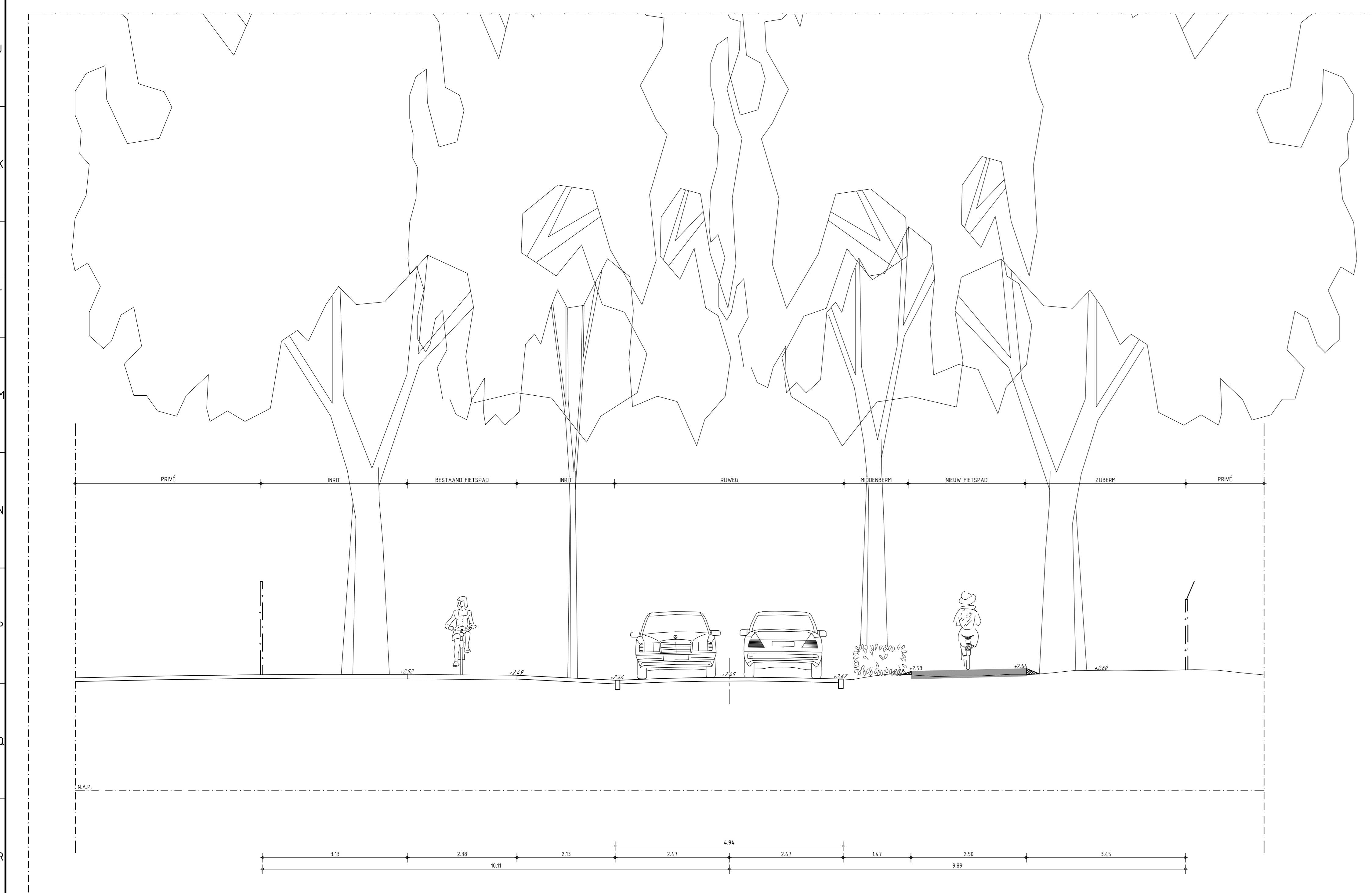
PRINCIEPE DOORSNEDE A-A (SCHAAL 1:50)
