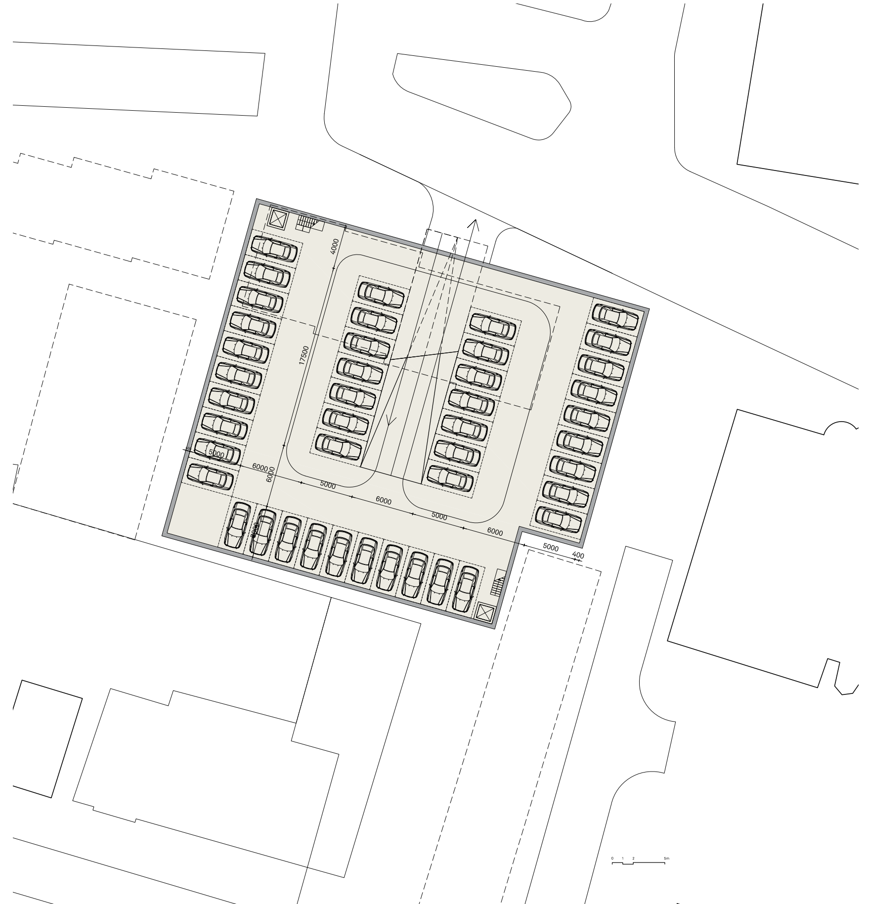
Parkeergarage met 43 parkeerplaatsen Met voldoende afstand van de bestaande bebouwing is er een parkeerbak geprojecteerd met verticale verbinding het Entreeplein en in Organic
